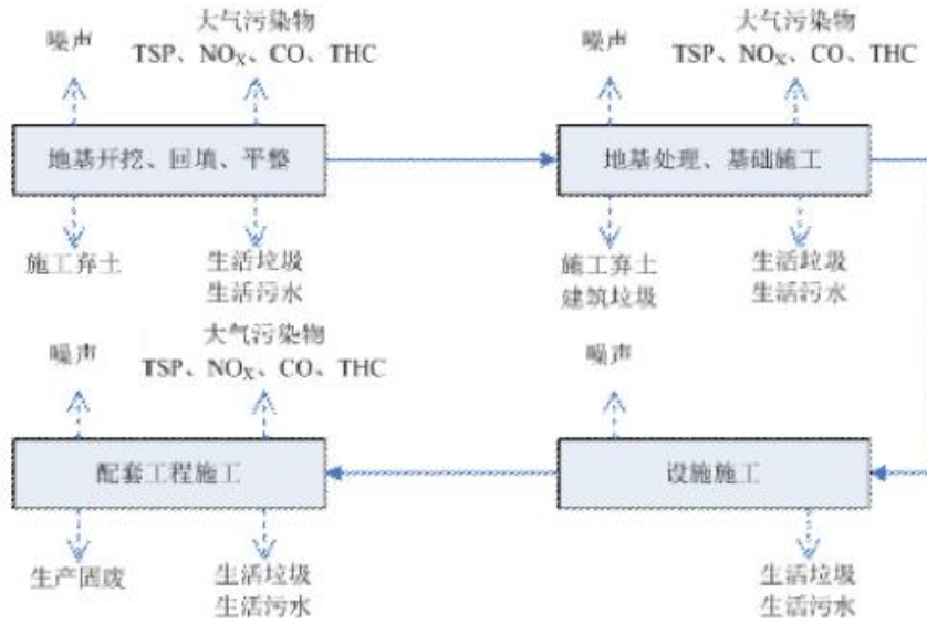
图 2.2.1 施工期主要流程及产污环节
