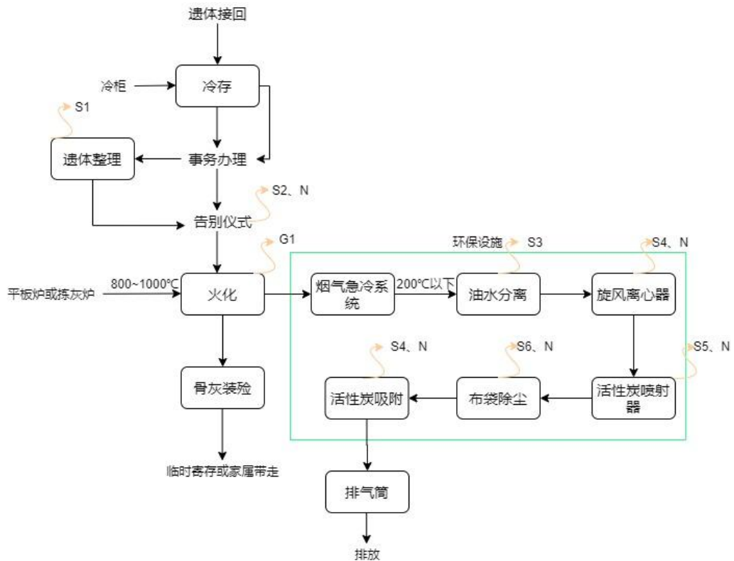
图 2.2.2 工艺流程及产污环节
