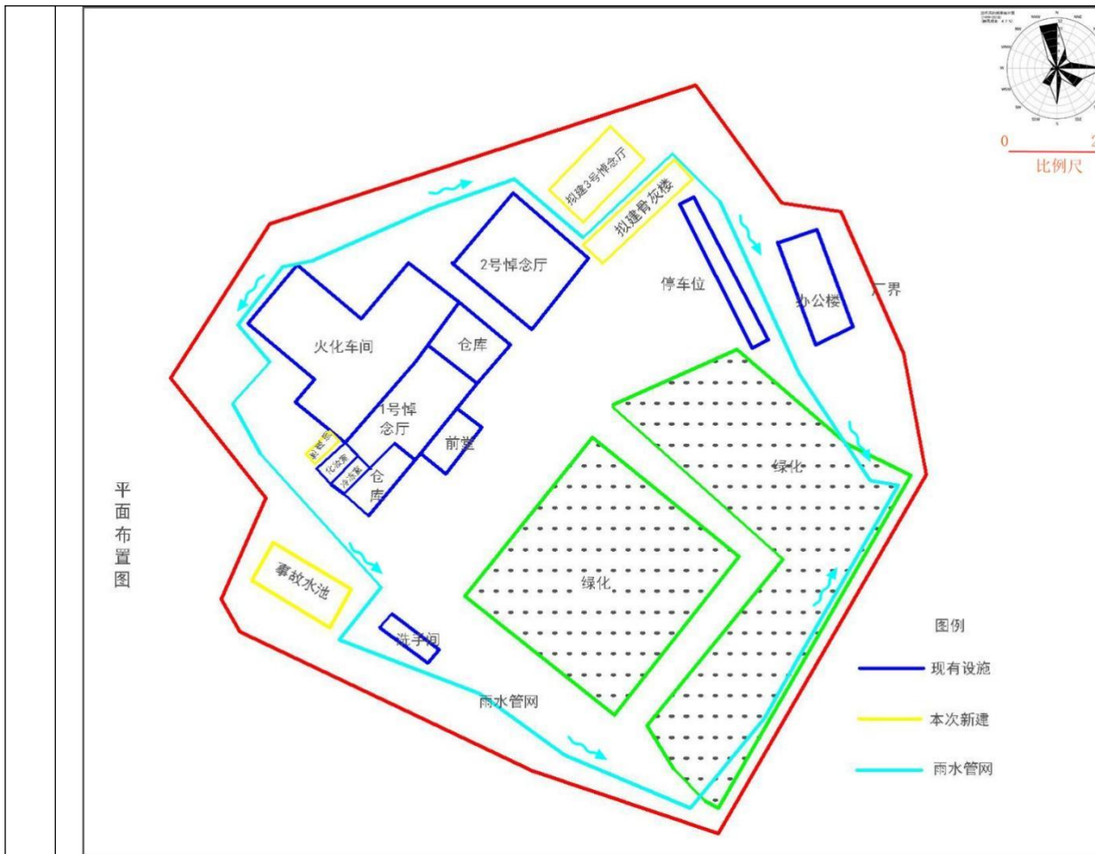
图 4-3 场内雨水管网及雨水流向图
